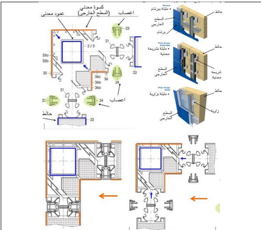
شكل (20.4): المرحلة الاولى والثانية والثالثة لطريقة تثبيت ألواح الالمنيوم .. وهنا الشكل عن اليمين يوضح تجميع الكسوة على العمود المعدني ومن ثم ربط الحائط بالقطاع المعدني في نفس الجانب وأيضا ربط الاعصاب بالسطح الخارجي لتقليل الفراغات، وعن اليسار الشكل النهائي للركن الخارجي. المصدر: الحلو، محمد: مقابلة شخصية، شركة الحلو للألمنيوم، 2014م.
