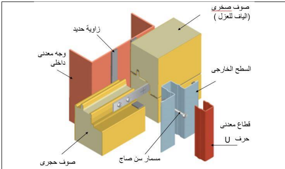
شكل (11.4): نظام تركيب ألواح الألمنيوم المركبة Composite Panel.
